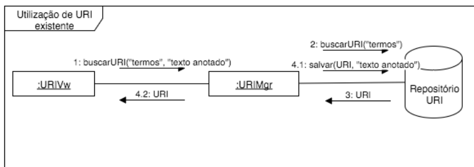
Figura 25: Busca e atualização de um identificador na base de dados
