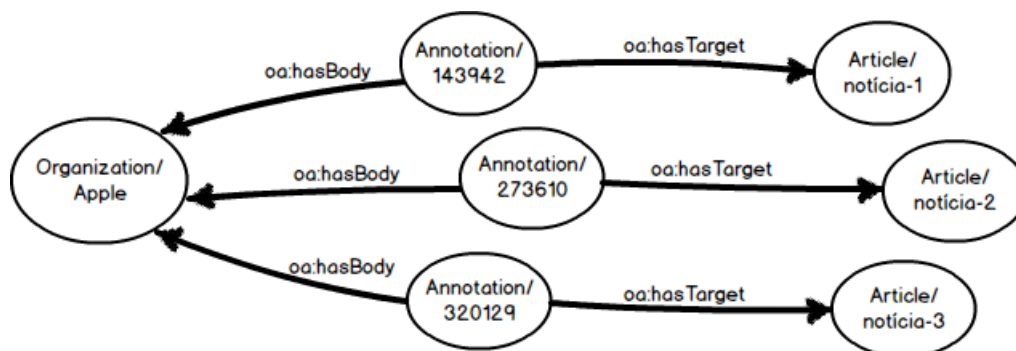
Figura 27: Grafo exibindo um recurso, suas anotações e as páginas onde aparece
