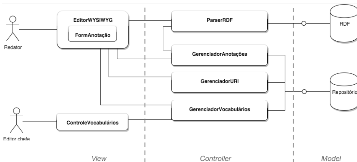
Figura 23: Esquema com os elementos que formam arquitetura da aplicação
