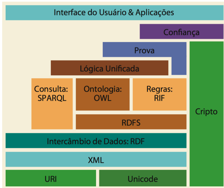
Figura 2: Conjunto de tecnologias da Web Semântica. Fonte: ISOTANI; BITTENCOURT (2015)
