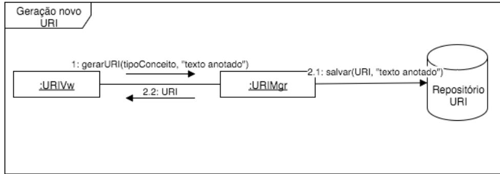
Figura 24: Geração de um URI novo
