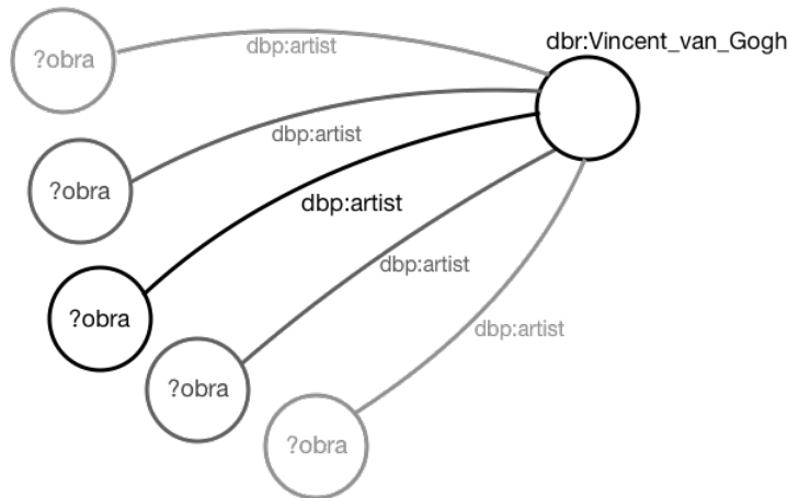
Figura 5: Representação de um grafo para uma consulta SPARQL
